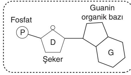
Guanin nükleotidi
