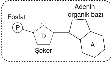
Adenin nükleotidi
